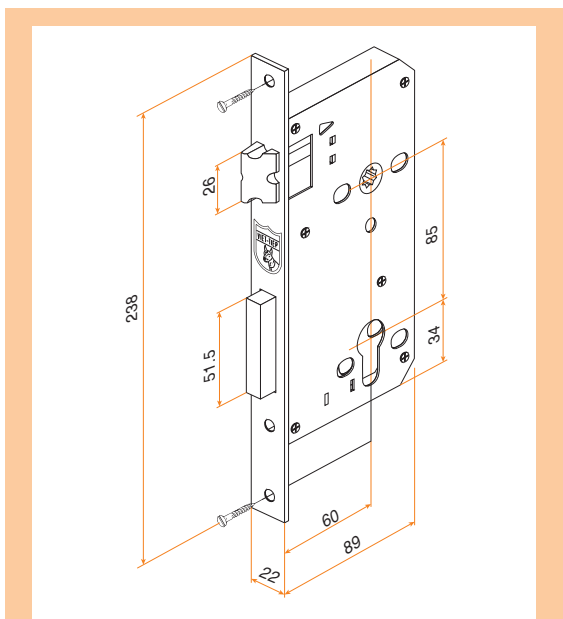
Hộp khóa 04292 Lock case 04292
