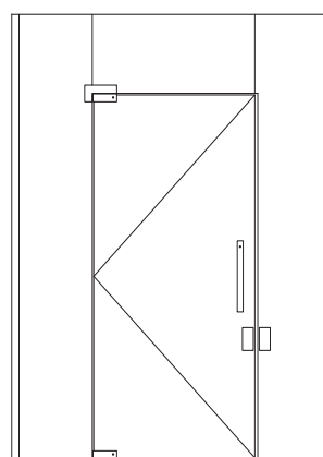
Bản lề thủy lực
